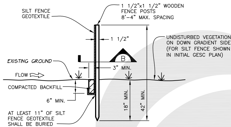
ELEVATION SCALE: 1" = 1'-0"
