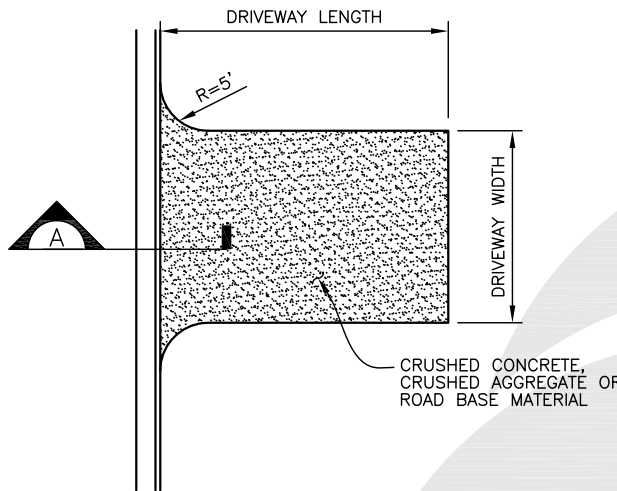
PLAN SCALE: 1" = 10'-0"
