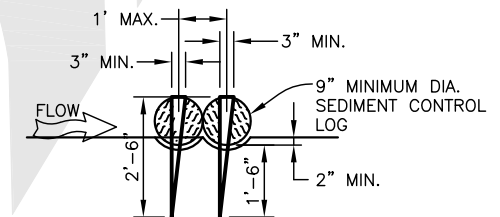
SECTION B SCALE: 1/2" = 1'-0"
