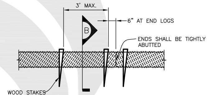
ELEVATION SCALE: 1/2" = 1'-0"
