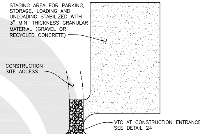
PLAN SCALE: 1" = 40'-0"
