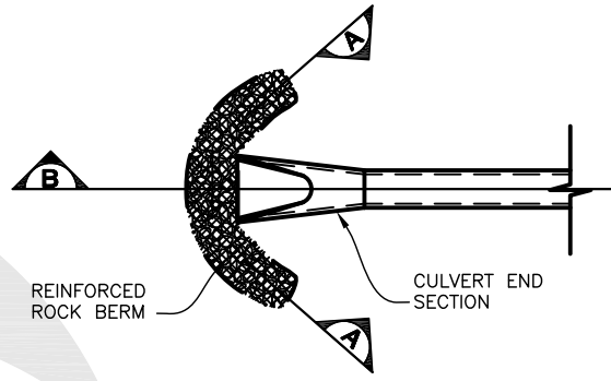
PLAN SCALE: 1" = 5'-0"
