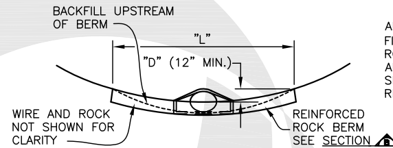
SECTION A SCALE: 1" = 5'-0"
